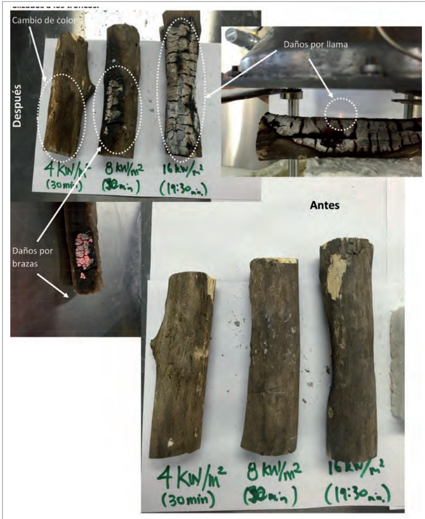
Figura 13. Tres muestras de troncos sometidos a 4 \text{ kW/m}^2 , 8 \text{ kW/m}^2 y 16 \text{ kW/m}^2 . El tronco calentado a 4 \text{ kW/m}^2 muestra los primeros indicios de degradación. Se puede observar el oscurecimiento del tronco pero no hay indicios de combustión. A 8 \text{ kW/m}^2 la combustión se inicia generando brazas pero no llama. A 16 \text{ kW/m}^2 se enciende una llama y se observa un consumo importante del tronco. Ensayos ejecutados el 20 y 21 de Julio del 2015.
